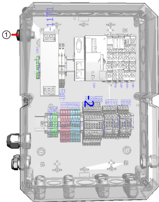
Figur 1. Matning styrskåp.
